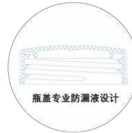
无密封圈设计，瓶盖瓶口倒角咬合
